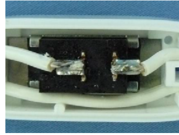
中間スイッチ内はんだ部
